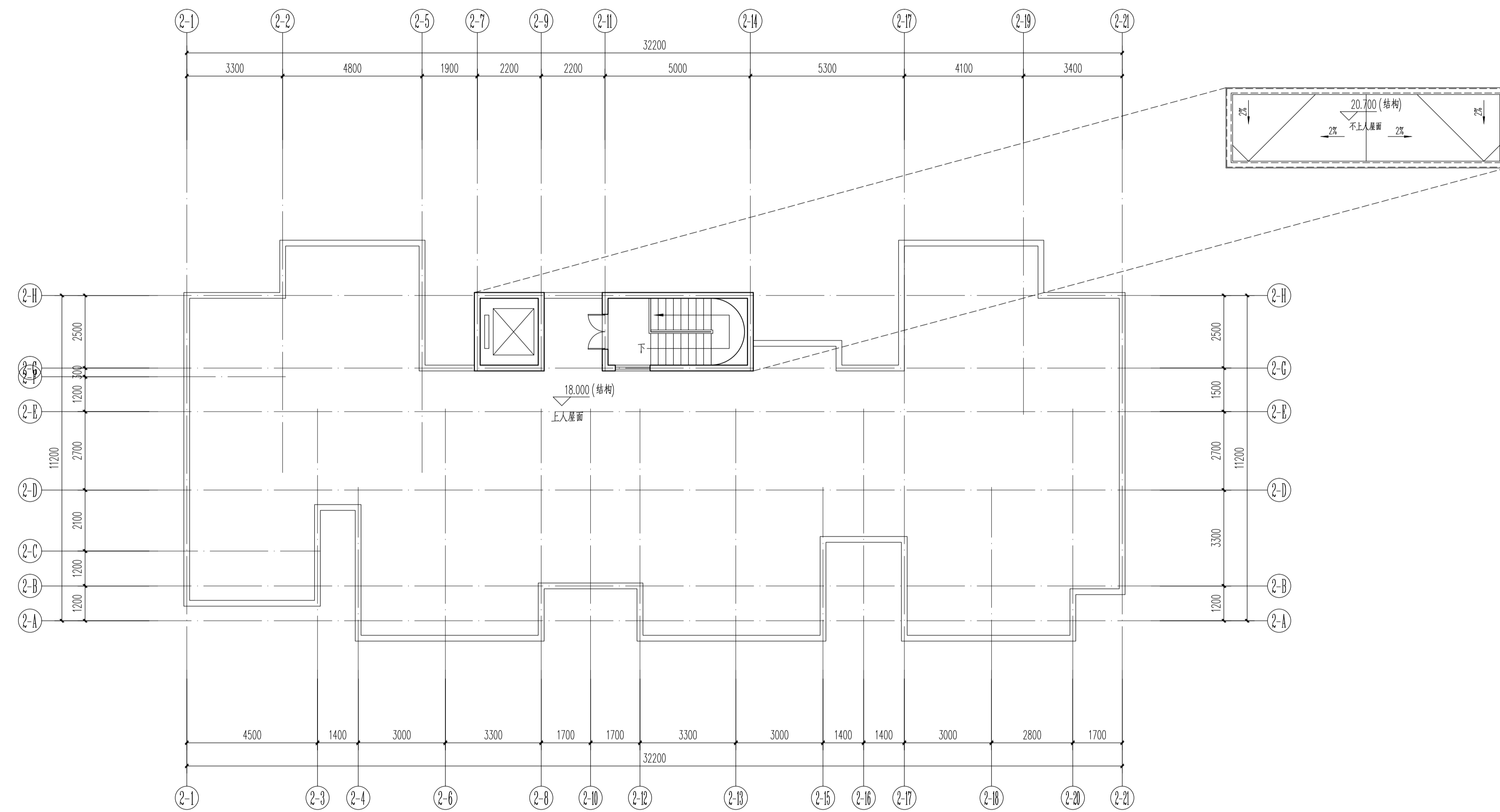
2#楼屋顶层平面图 1:100
