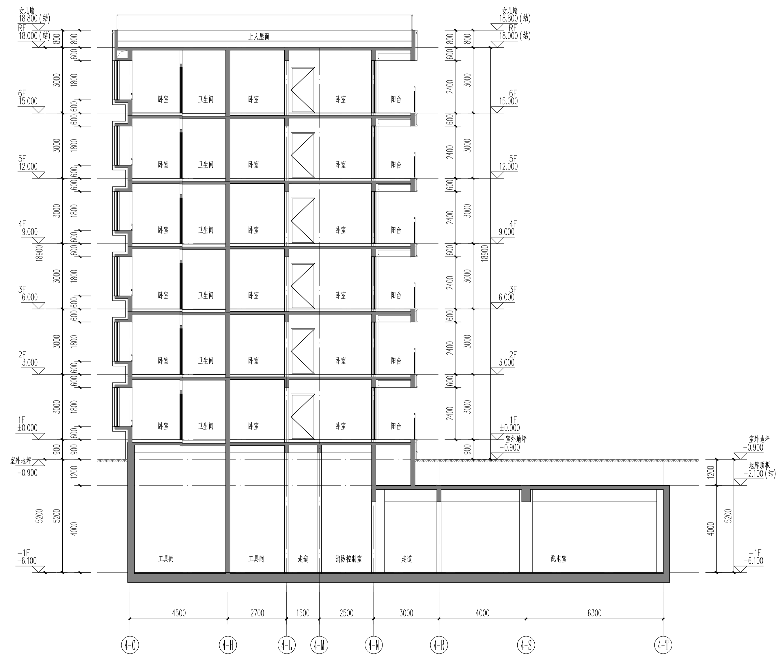
4#楼1-1剖面图 1:100
