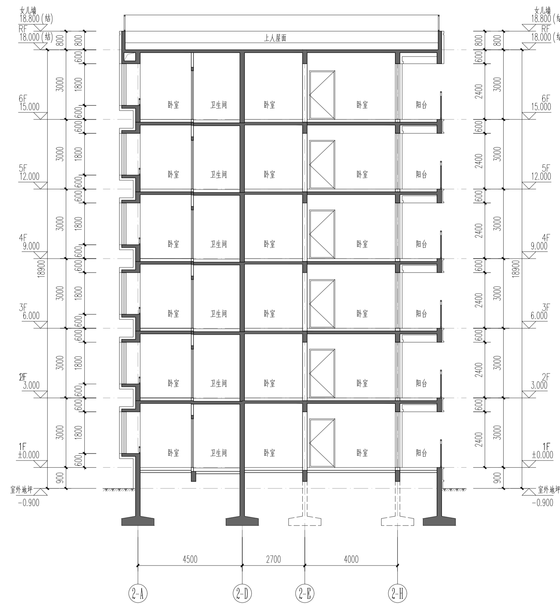
2#楼1-1剖面图 1:100
