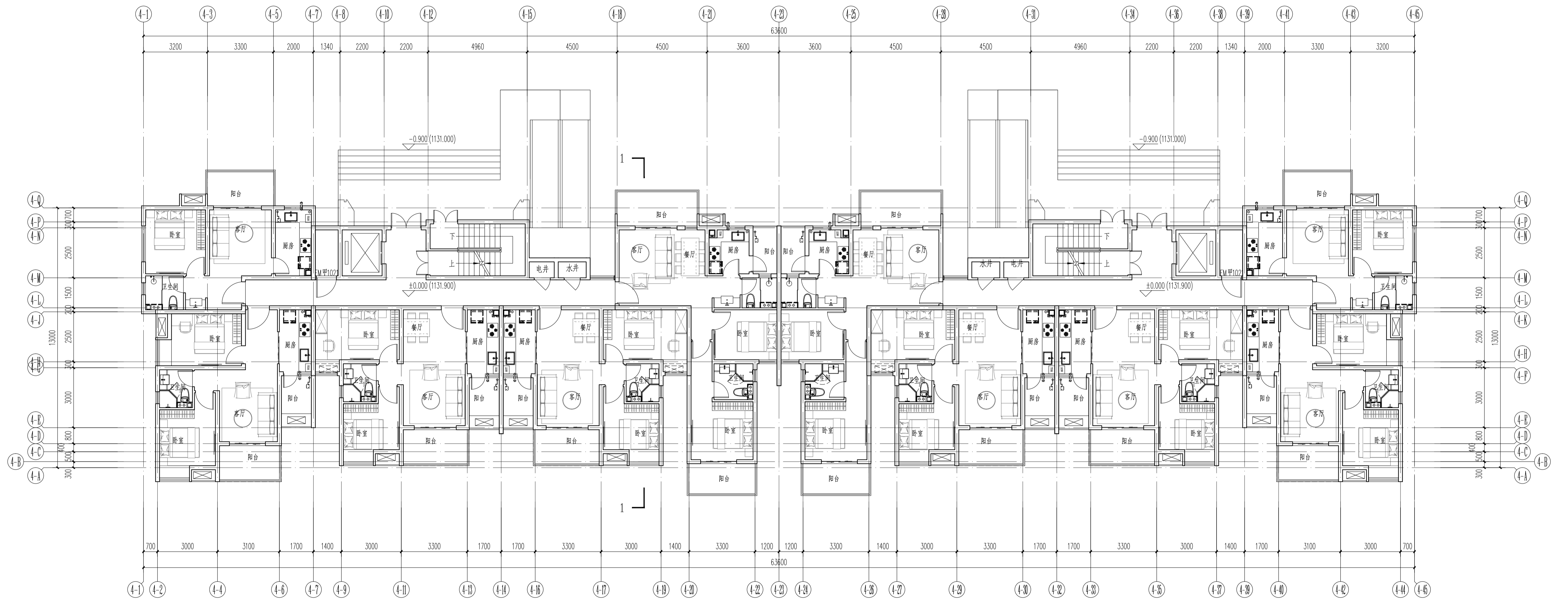
4#楼首层平面图 1:100
