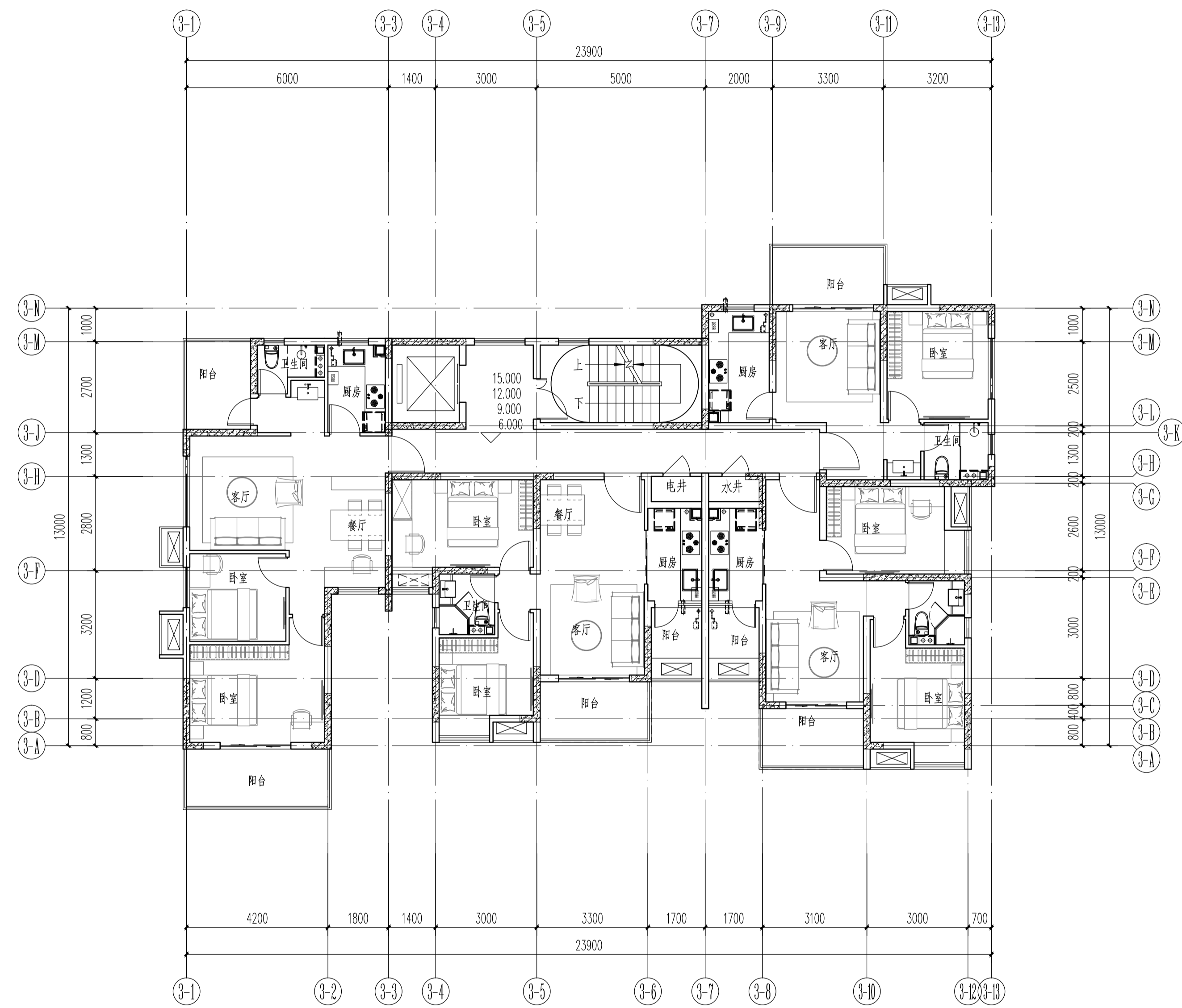
3#楼三至六层平面图 1:100
