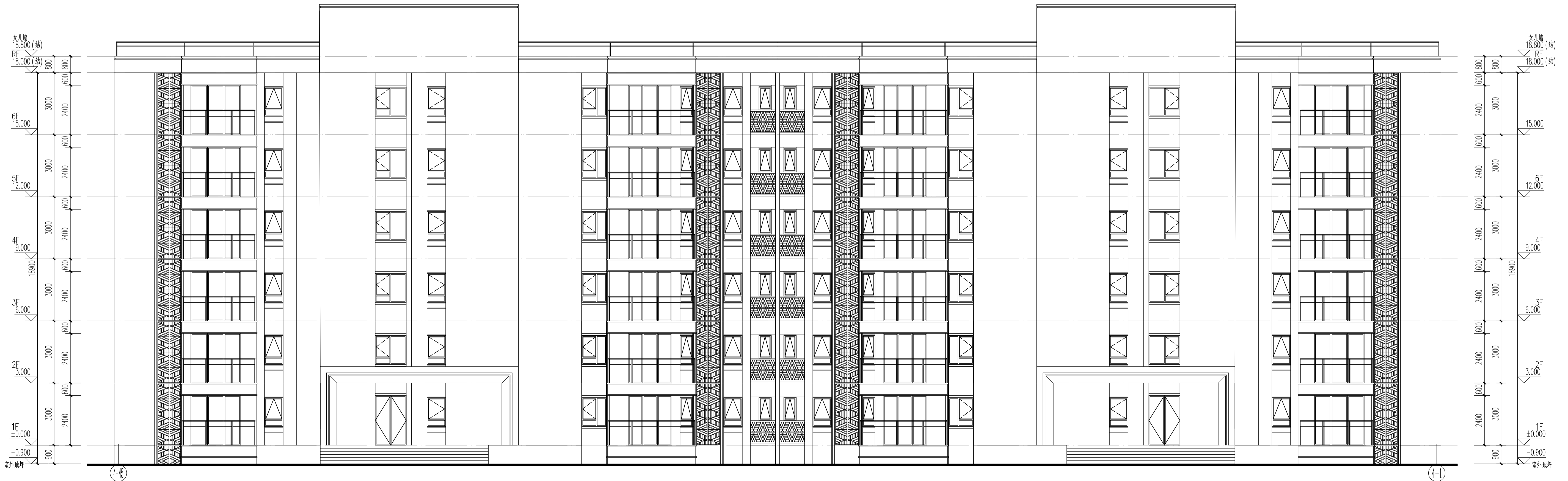
4#楼⑥至①立面图 1:100
