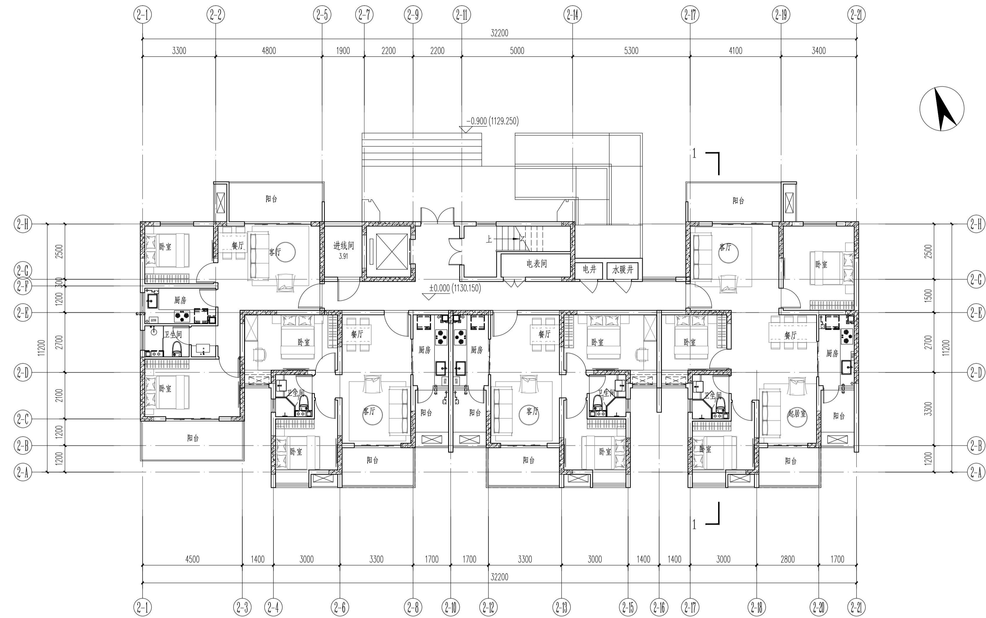
2#楼首层平面图 1:100
