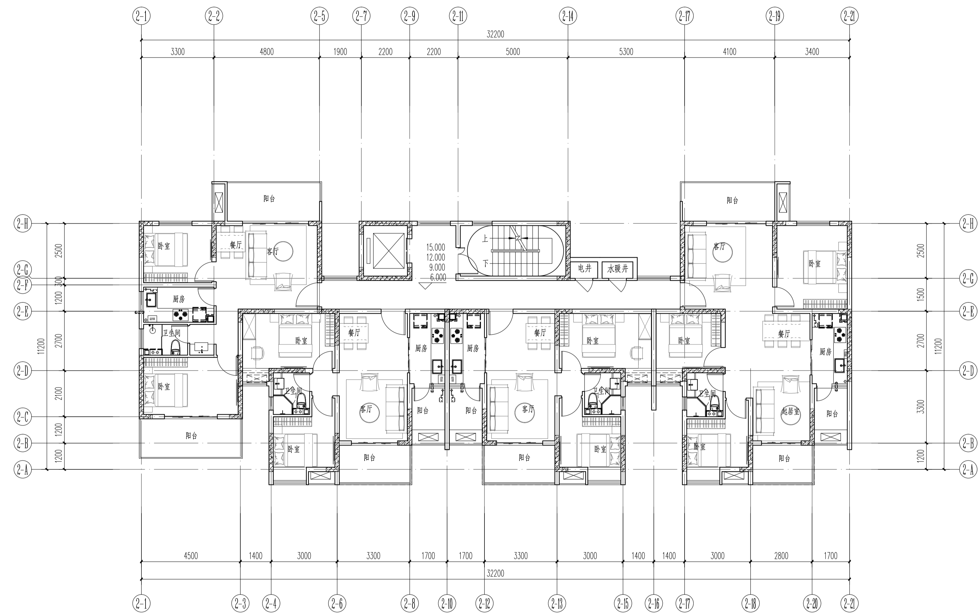
2#楼三至六层平面图 1:100
