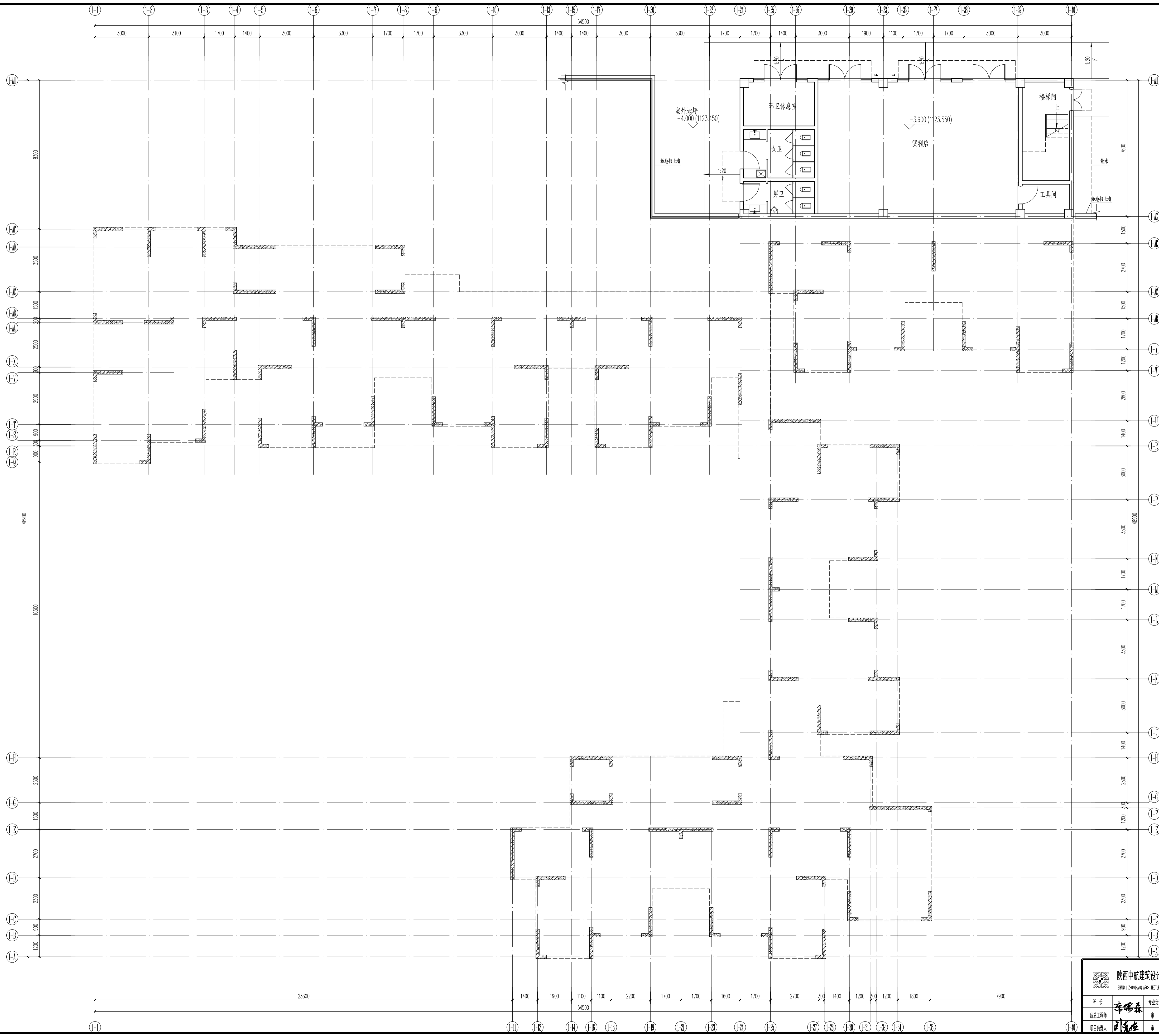
1#楼标高-3.900处平面图 1:100
