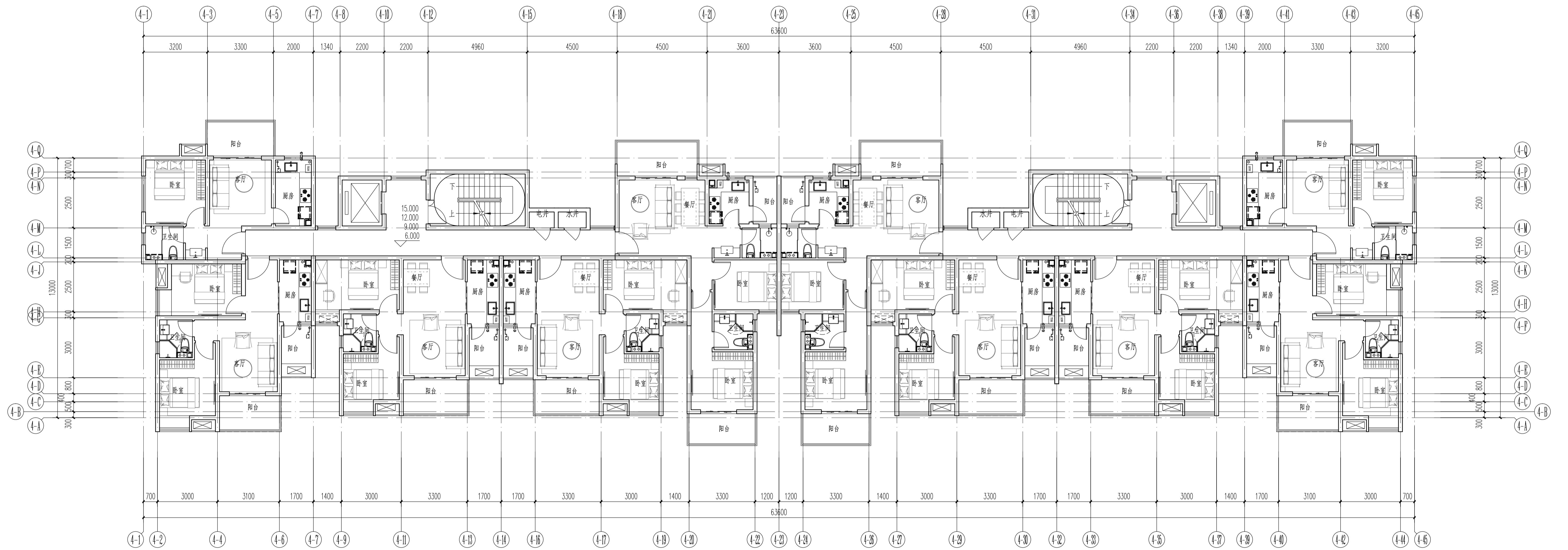
4#楼三至六层平面图 1:100
