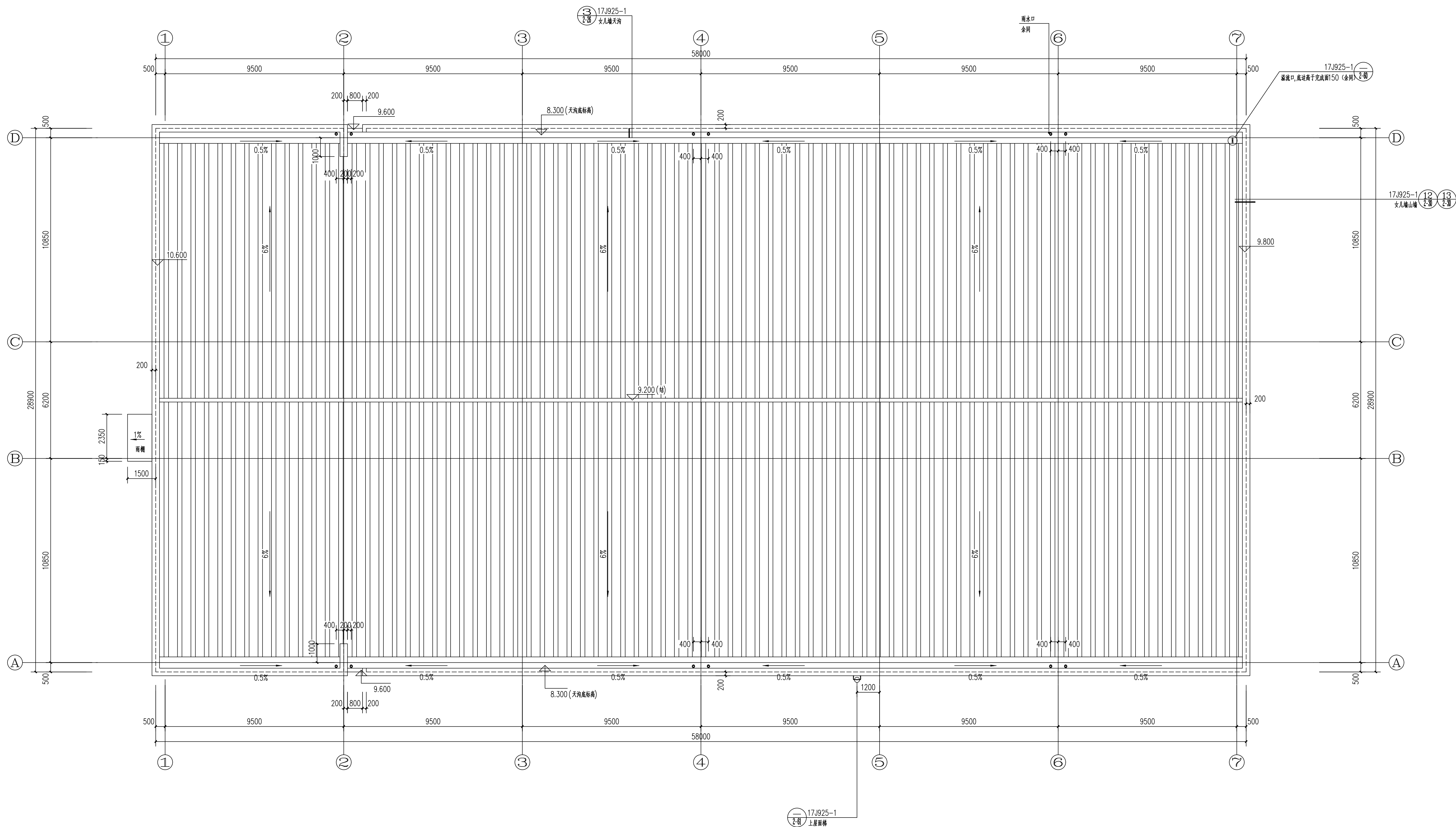
屋顶层平面图 1:100
