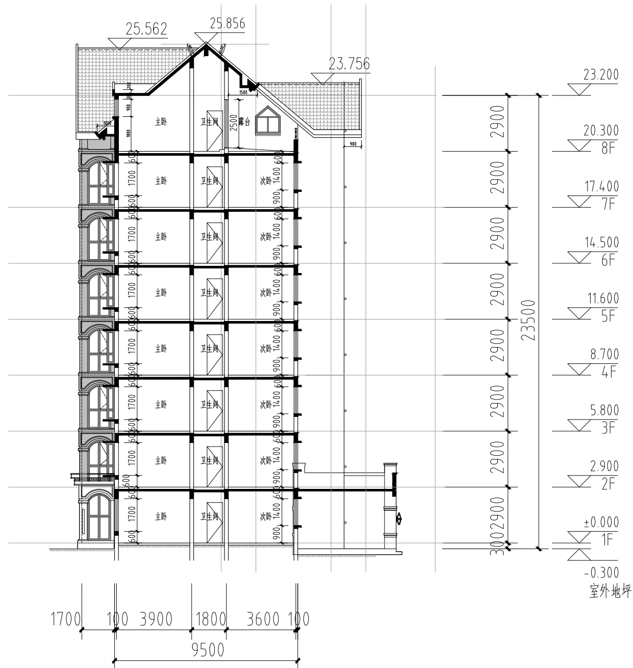
2-2 剖面图 1:200
