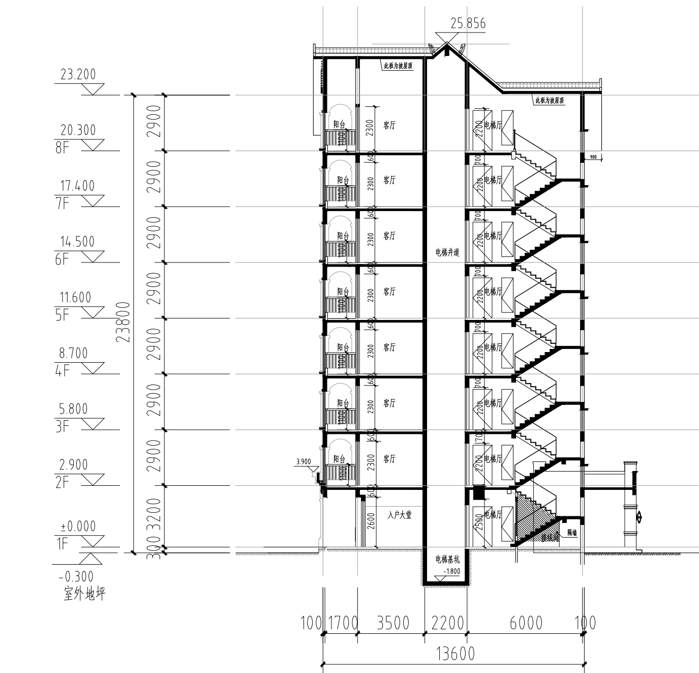
1-1 剖面图 1:200
