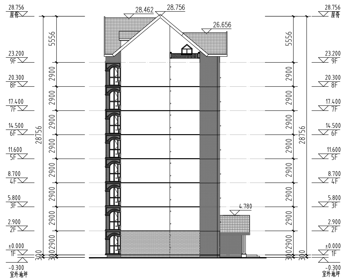
东立面图 1:200
