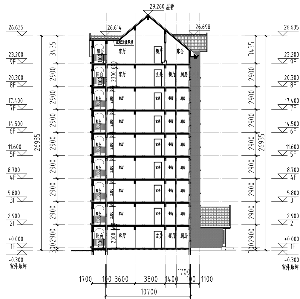
I—I 剖面图 1:200
