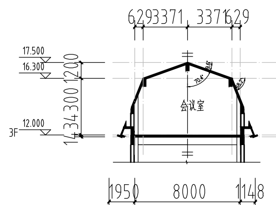
1~1剖面图 1:200
