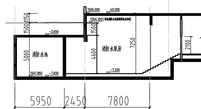
A-A剖面图 1:200
