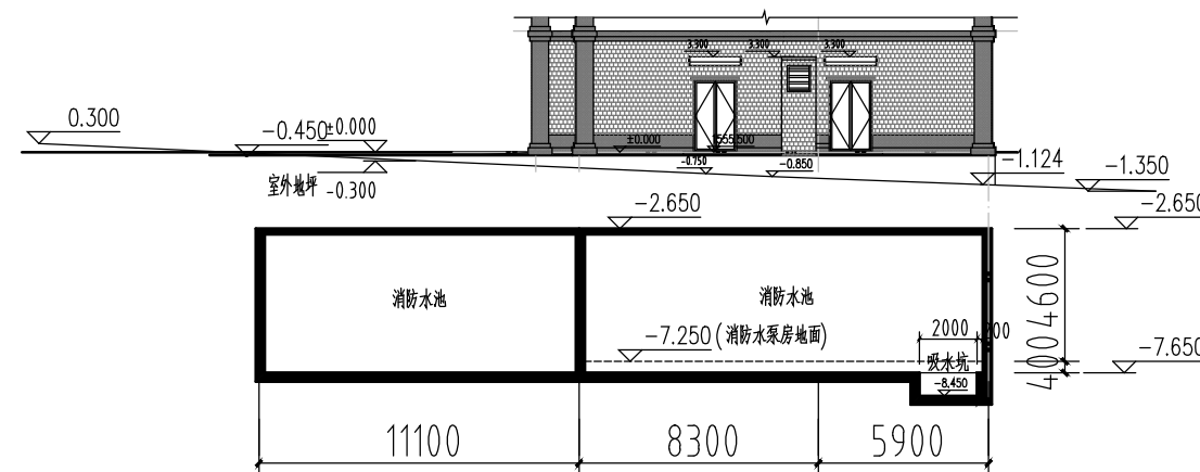
B-B剖面图 1:100
