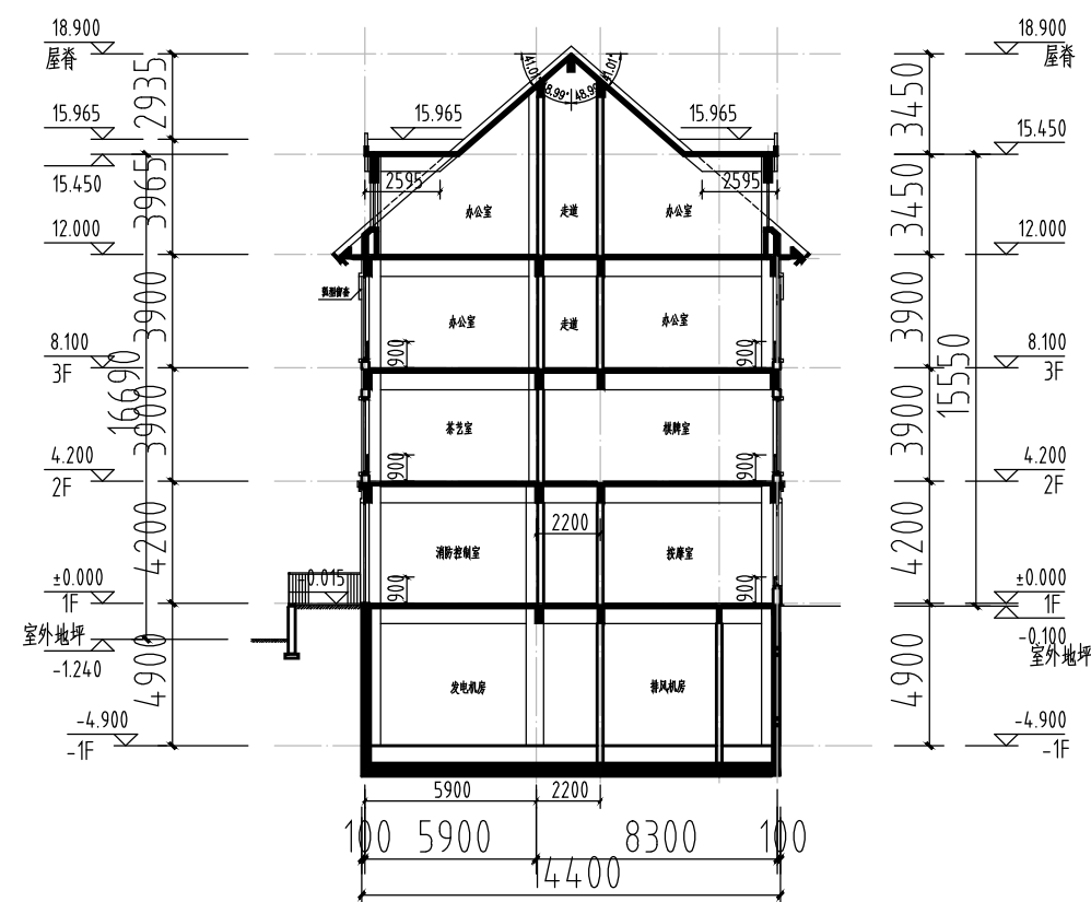
I - I 剖面图 1:200
