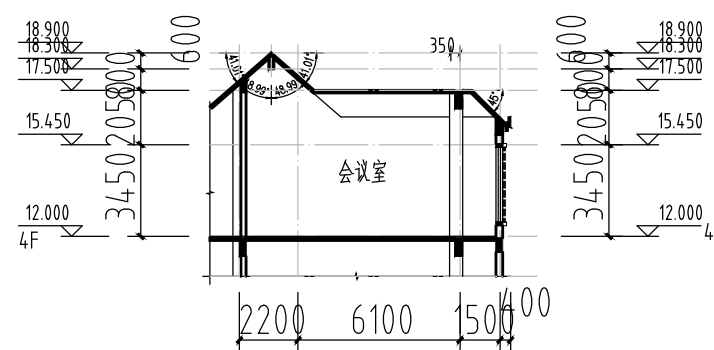
2~2剖面图 1:200
