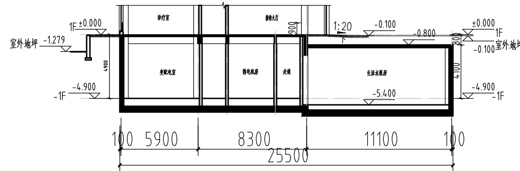
II-II 剖面图 1:200
