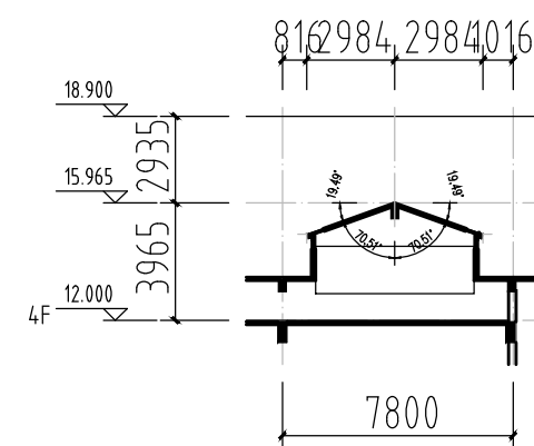
3~3剖面图 1:200
