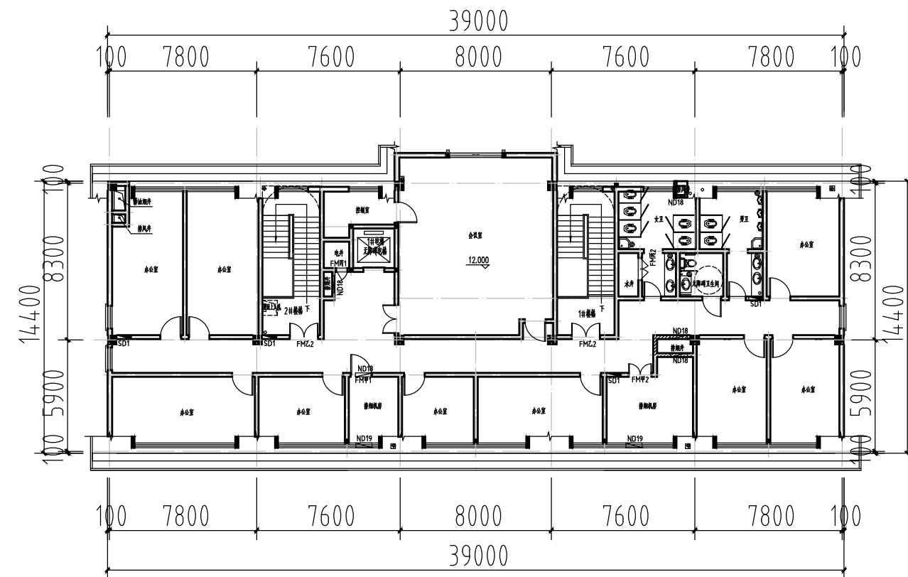
四层平面图 1:200
