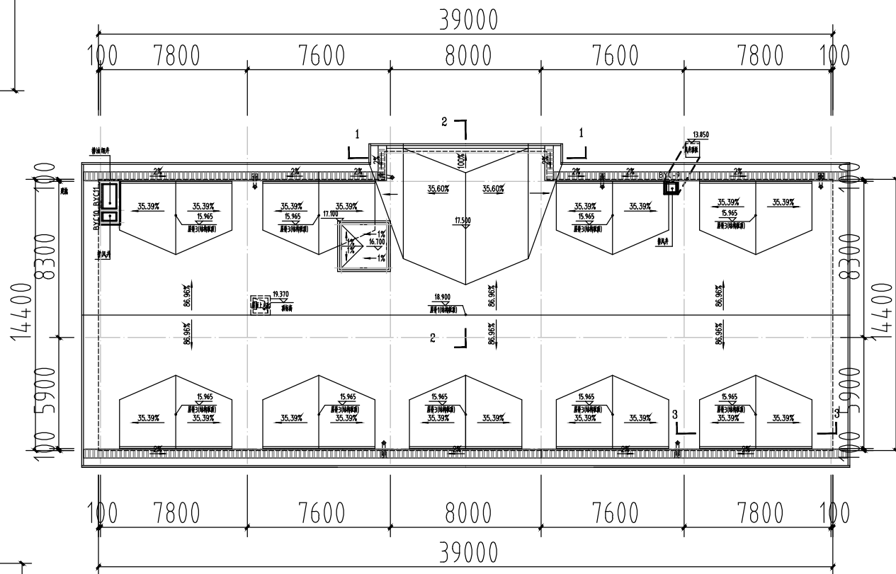
屋面平面图 1:200
