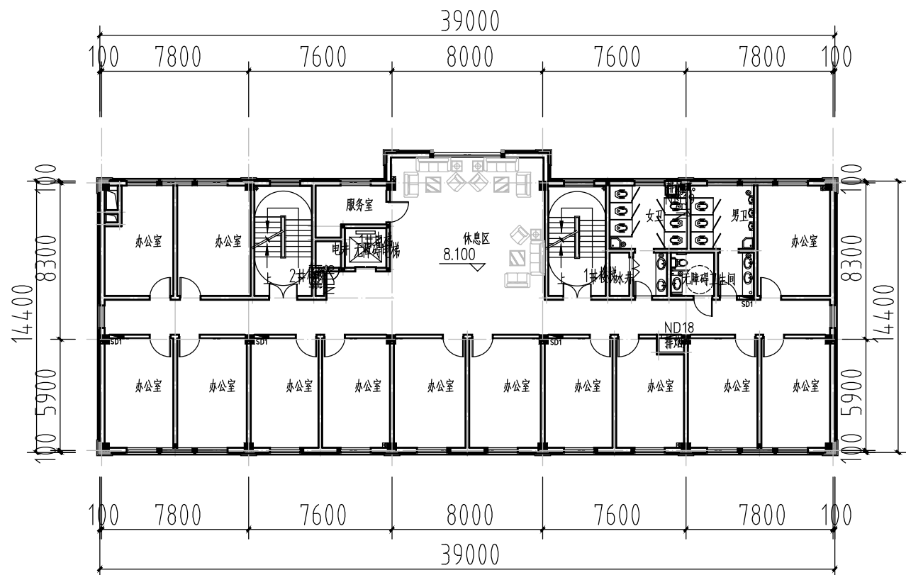
三层平面图 1:200
