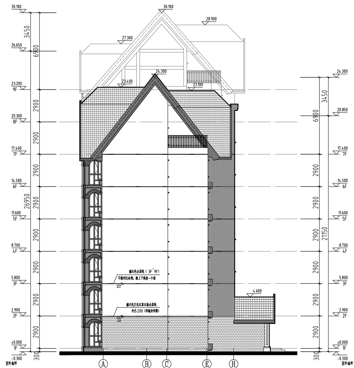
东立面图 1:200
