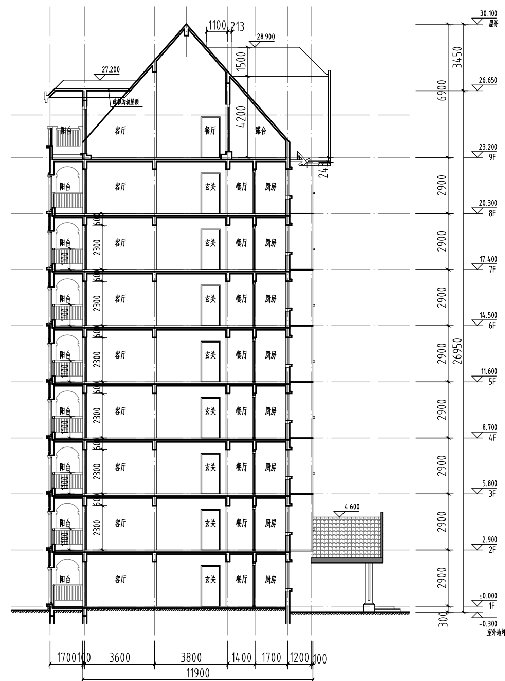
I—I 剖面图 1:200
