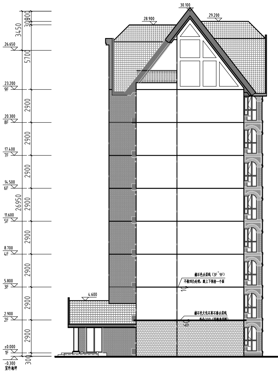
西立面图 1:200
