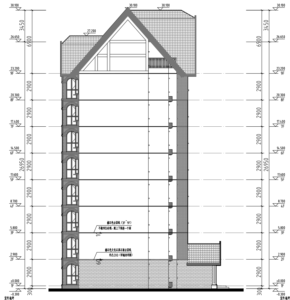
东立面图 1:200
