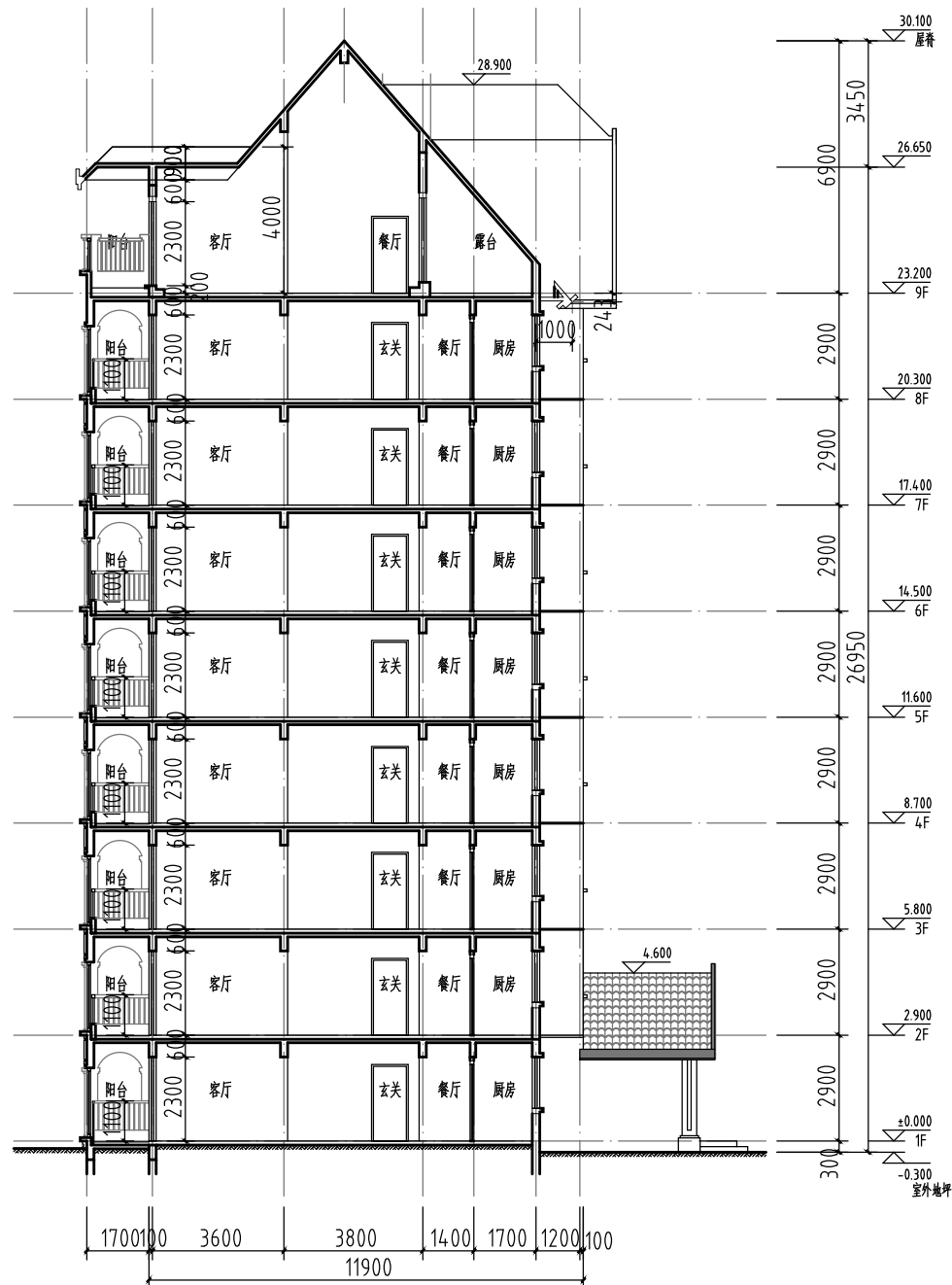
I ~ I 剖面图 1:200
