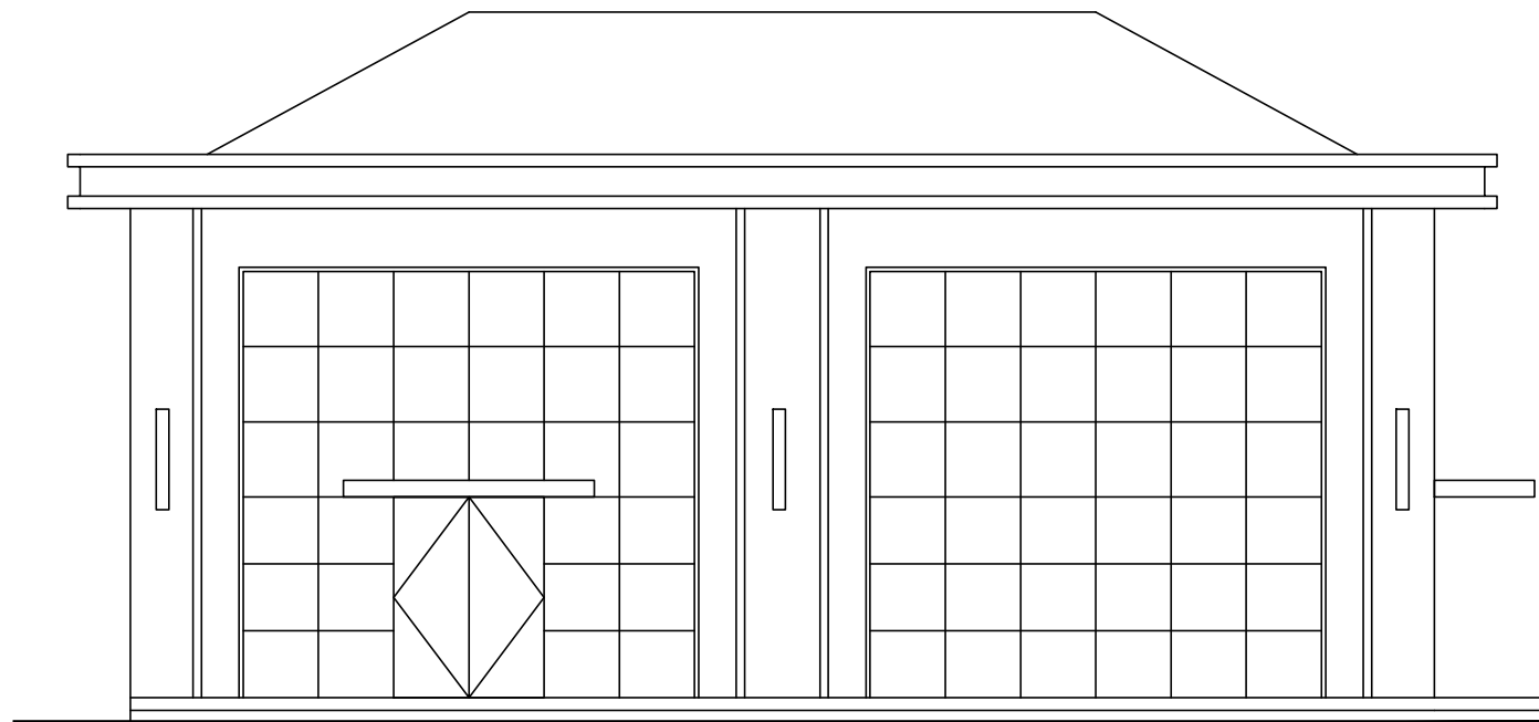
南立面图 1:100
