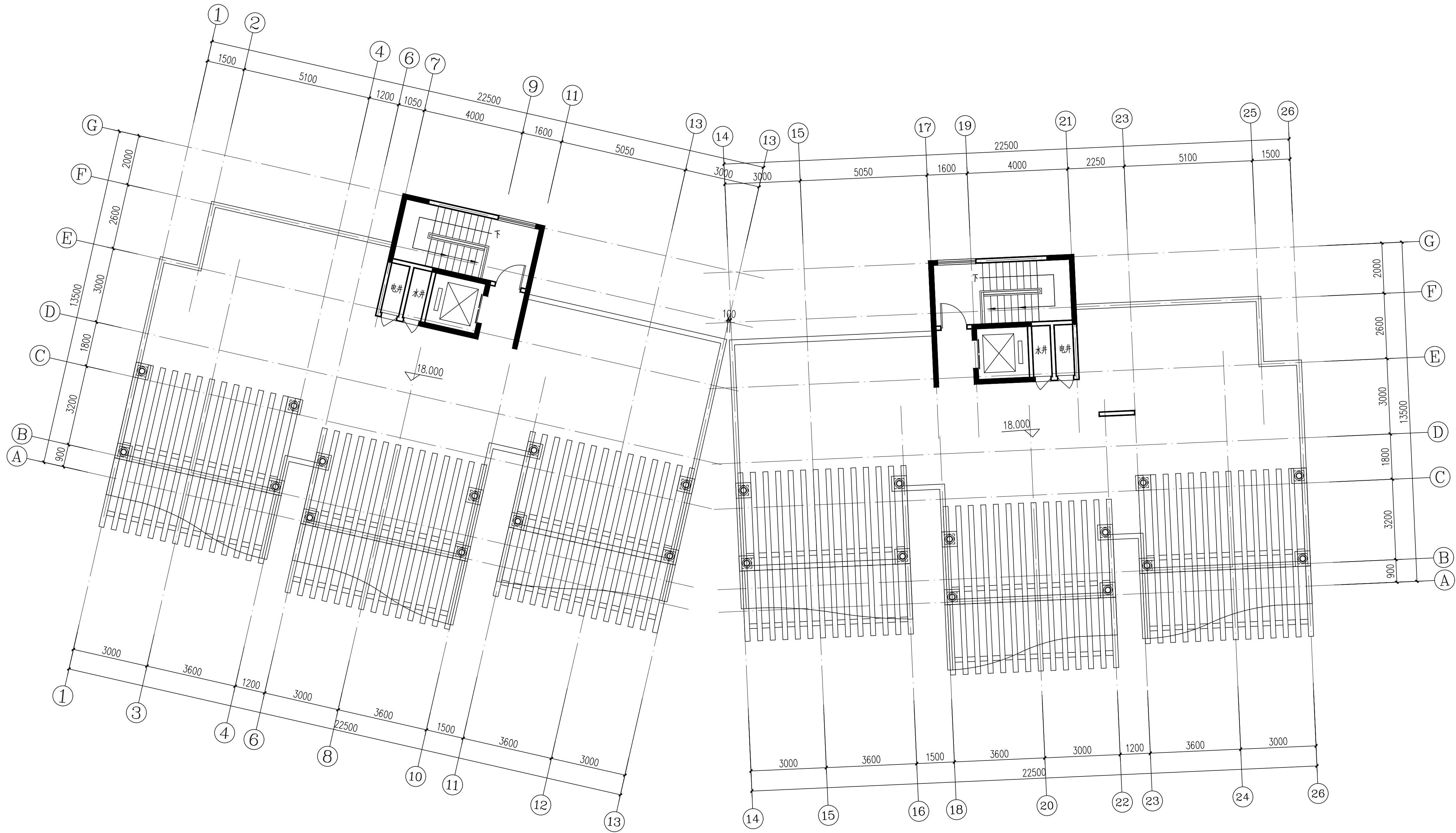
屋面平面 1:100
