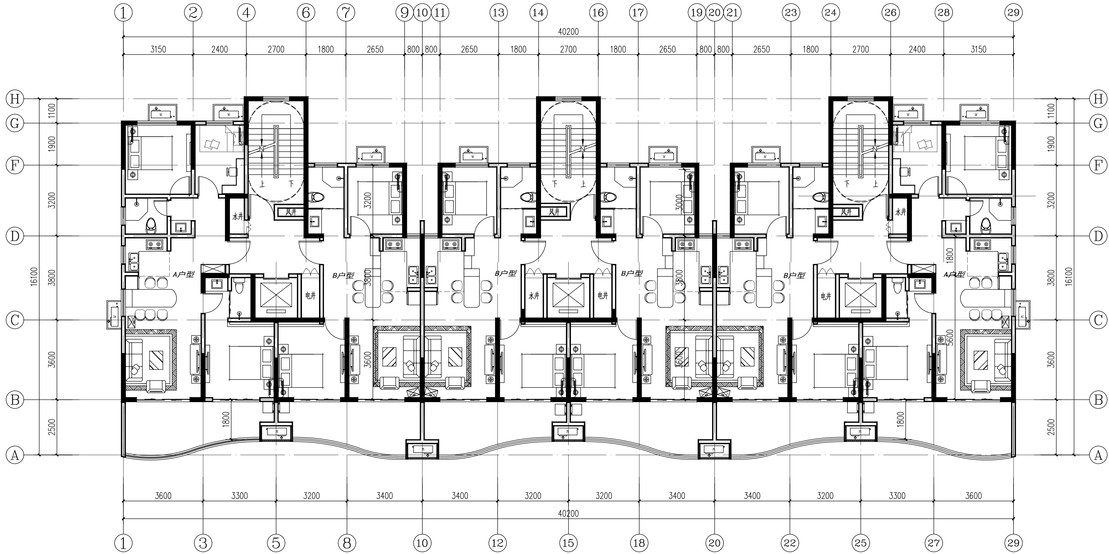
二~十三层平面 1:100
