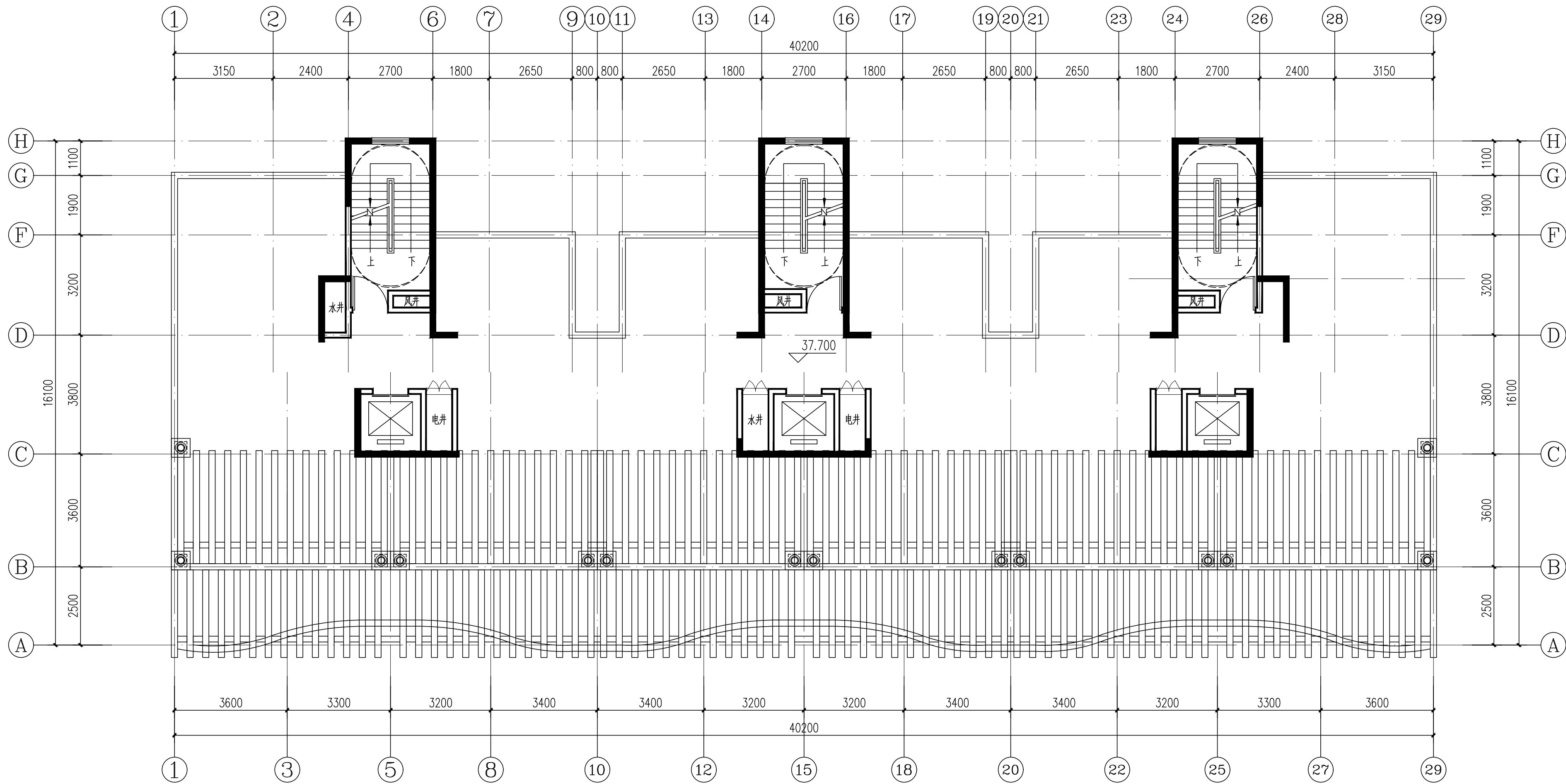
屋面平面 1:100
