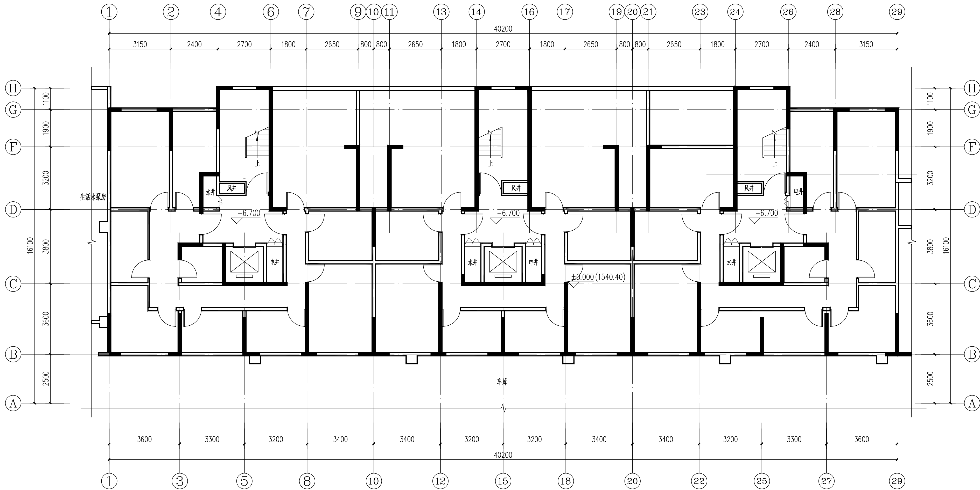
地下一层平面 1:100
