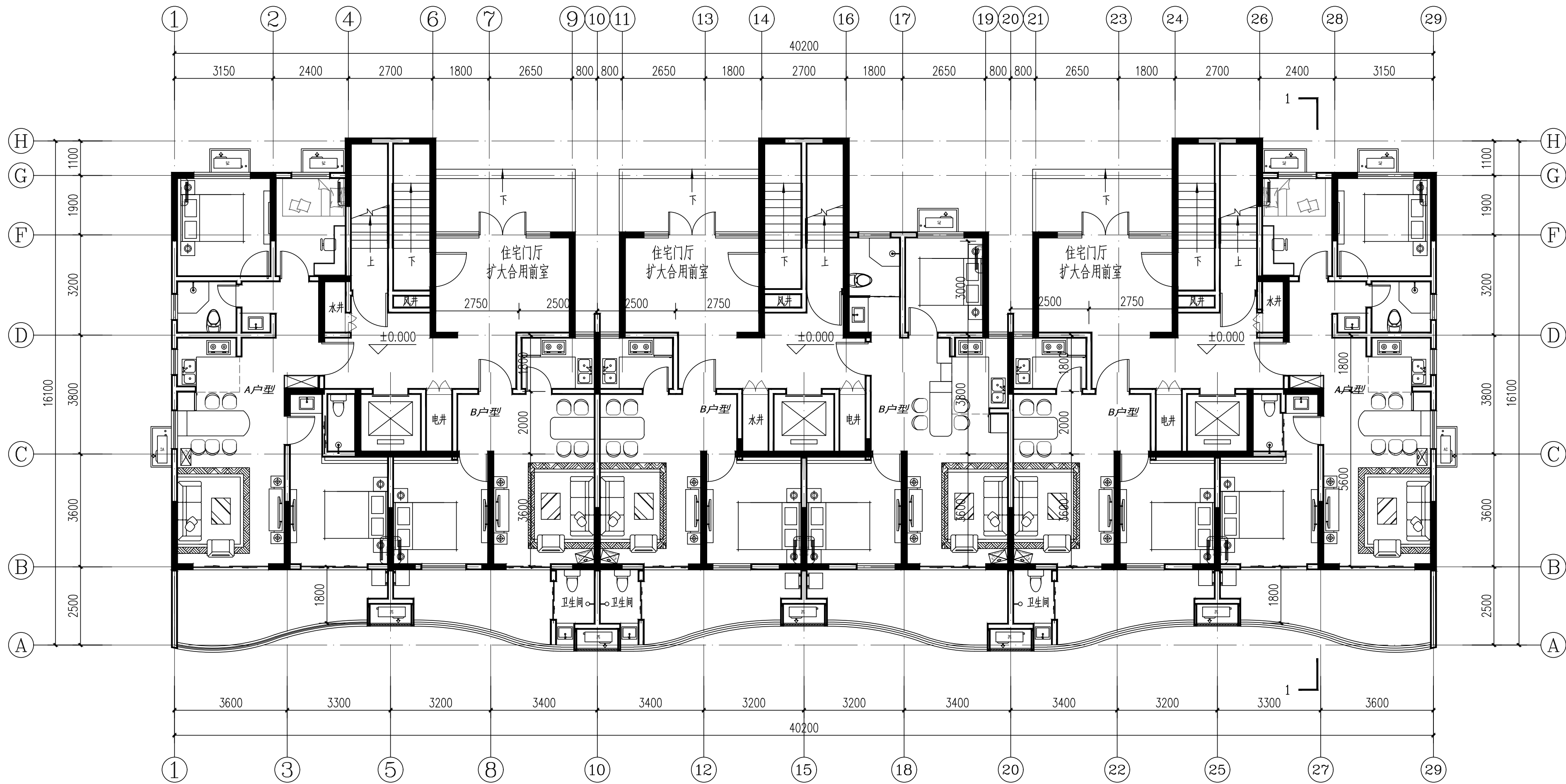
一层平面 1:100
