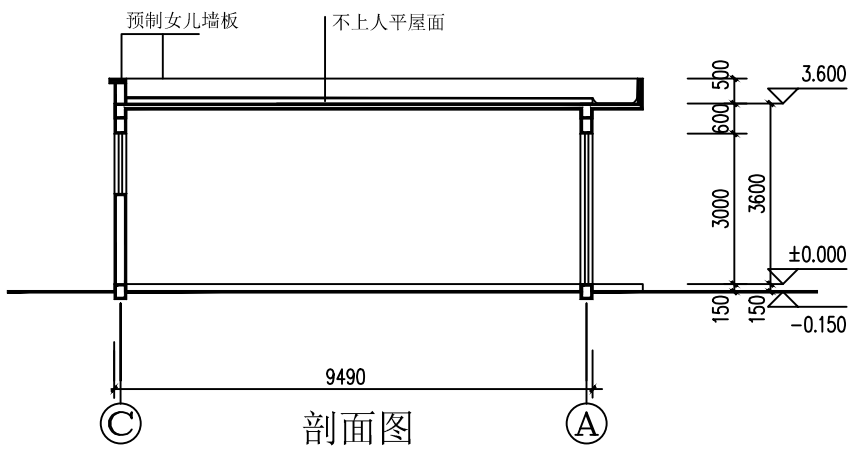
南立面图 1:100
