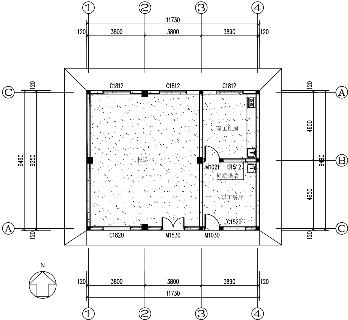
底层平面图 1:100
