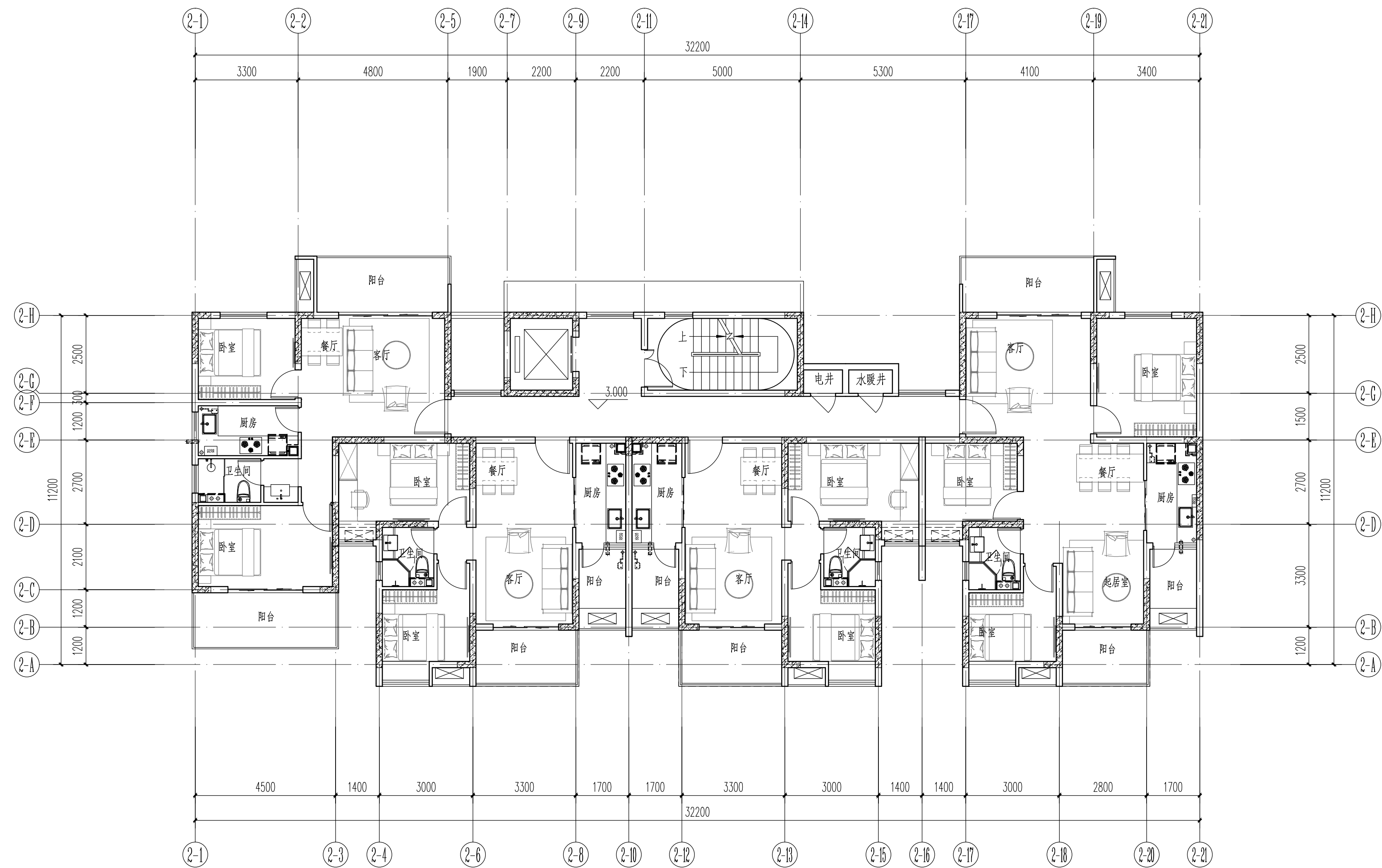
2#楼二层平面图 1:100
